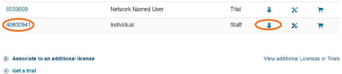
Şekil 1: Hesaba giriş
