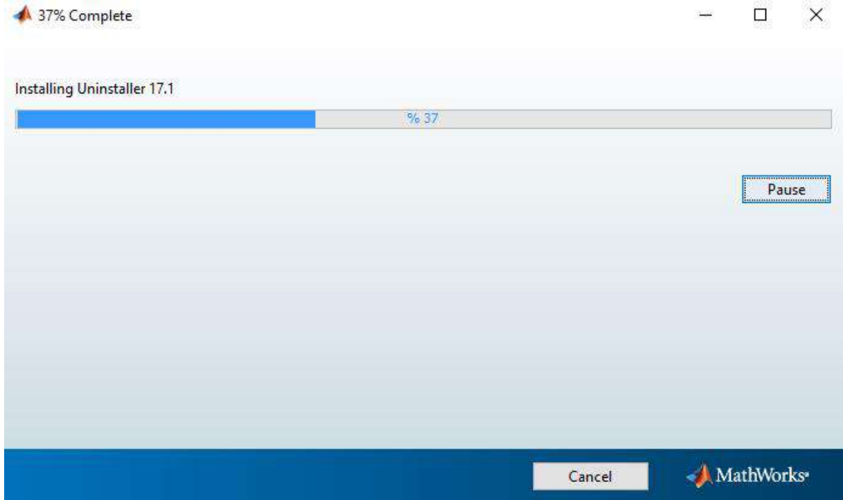
Şekil 17: Yükleme süreci
