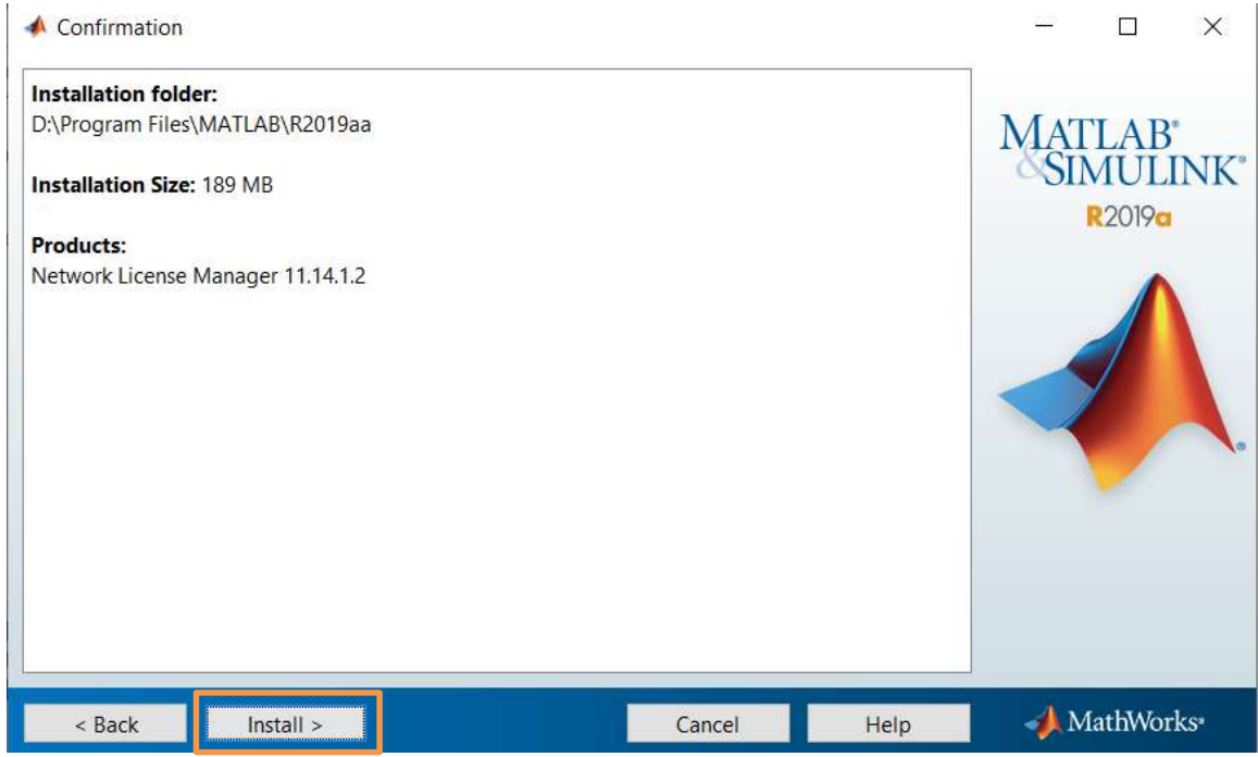
Şekil 16: Doğrulama Ekranı
