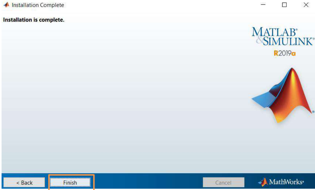
Şekil 21: Yükleme tamamlandı
