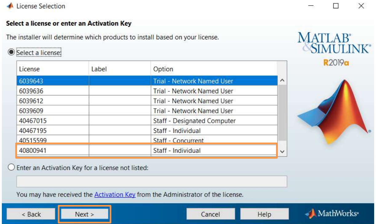
Şekil 15: Toolboxların seçilimi
